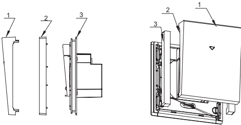
Рисунок 3 – Порядок монтажа выключателя / Figure 3 – Switch installation procedure / 3 сурет – Ажыратқышты монтаждау тәртібі / Figura 3 – Procedura de instalare a întreruptorului / 3-rasm – Viklyuchatelni montaj qilish tartibi
