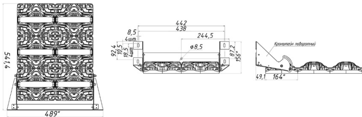
Рисунок 1 Общий вид светильника «L-pixel 6 banner» Поворотное крепление
