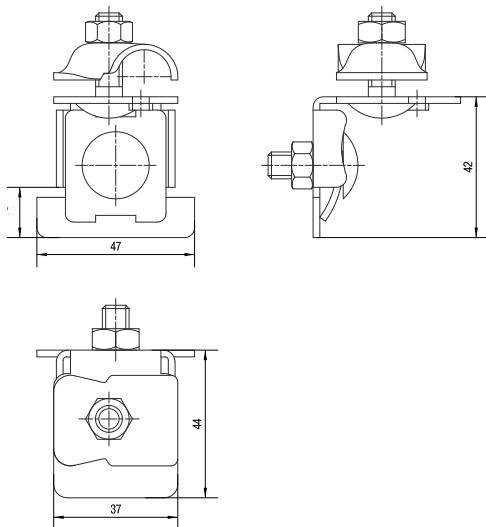
Рисунок 1 – Габаритные размеры
