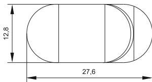
1 – изделие / product; 2 – клейкая лента / adhesive tape KC-1 / KS-1
