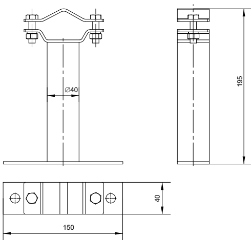
Рисунок / Figure 1 – Габаритные размеры / Overall dimensions
