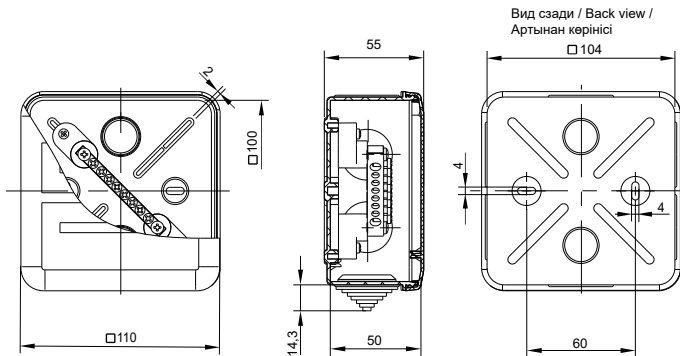
Рисунок / Figure / Сурет 2 – Коробка / Box / Қорабы КУП КМ41361
