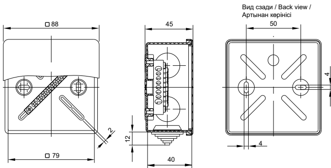
Рисунок / Figure / Сурет 1 – Коробка / Box / Қорабы КУП КМ41360
