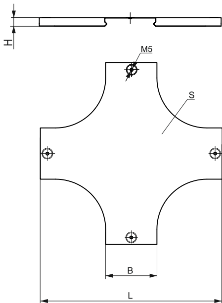
Рисунок 1 – Крышка крестовины плавной серии ESCA
