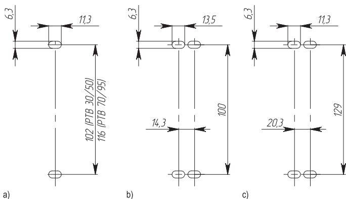
Рисунок / Figure 2 – а) установочные размеры клемм PTB35/50SH и PTB70/95SH, б) установочные размеры клеммы PTB120/150SH, в) установочные размеры клемм PTB185/240SH и PTB300SH / а) mounting dimensions of PTB35/50SH and PTB70/95SH terminals, б) mounting dimensions of PTB120/150SH terminals, в) mounting dimensions of PTB185/240SH and PTB300SH terminals
