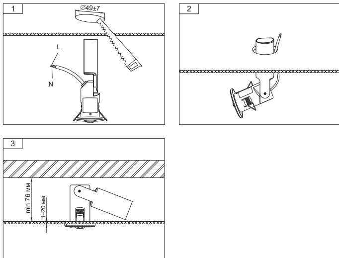
Рисунок 6 – Монтаж ДПА 060
