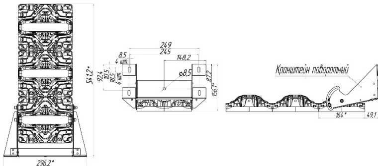
Рисунок 1 Общий вид светильника «L-pixel 3 banner» Поворотное крепление
