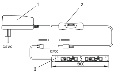
Рисунок 13 – Подключение LSR1-1-060-20-1-2XD12-S3
