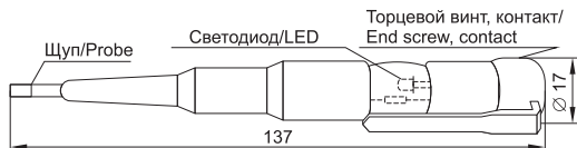
Рисунок 1 - Габаритные размеры пробника / Figure1 - Overall dimensions of tester
