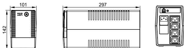
Рисунок 2 – Внешний вид ИБП типа EST-650VA-1-001-L, EST-850VA-1-001-L, EST-1000VA-1-001-L
