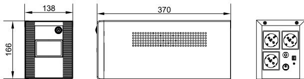
Рисунок 9 – Внешний вид ИБП типа EST-1200VA-1-002-S
