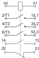
Рисунок 7 – Схема электрическая КМИе-34012 ÷ КМИе-49512 / Figure 7 – Electric diagram КМIе-34012 ÷ КМIе-49512 / 7 сурет – КМИе-34012 ÷ КМИе-49512 электрлі схемасы
