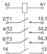
Рисунок 5 – Схема электрическая КМИе-10910 ÷ КМИе-23210 / Figure 5 – Electric diagram КМIе-10910 ÷ КМIе-23210 / 5 сурет – КМИе-10910 ÷ КМИе-23210 электрлі схемасы
