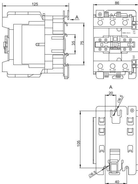
Рисунок 4 – Габаритные и установочные размеры КМИе-48012, КМИе-49512 / Figure 4 – Overall and mounting dimensions КМИе-48012, КМИе-49512 / 4 сурет – КМИе-48012, КМИе-49512 габариттік және орнату өлшемдері
