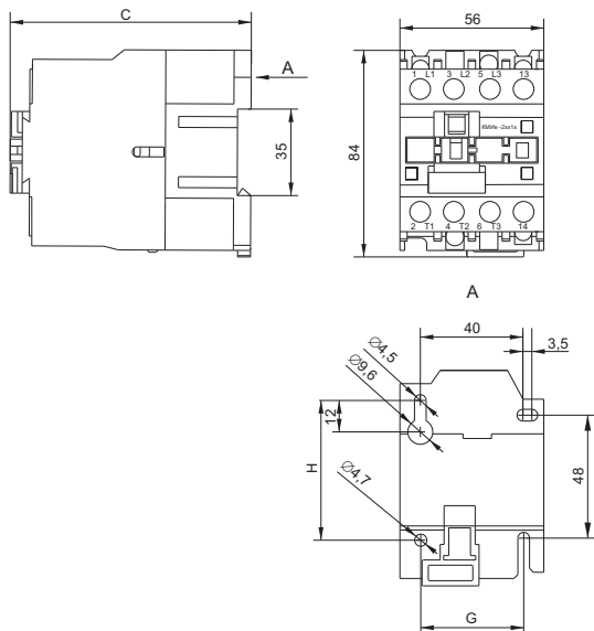
Рисунок 2 – Габаритные и установочные размеры КМИе-2321(0/1), КМИе-2251(0/1) / Figure 2 – Overall and mounting dimensions KMIe-2321(0/1), KMIe-2251(0/1) / 2 сурет – КМИе-2321(0/1), КМИе-2251(0/1) габариттік және орнату өлшемдері
