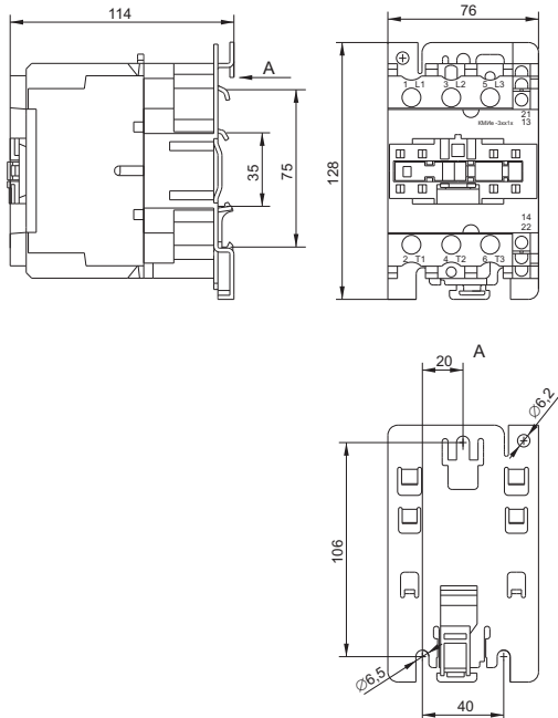
Рисунок 3 – Габаритные и установочные размеры КМИе-34012, КМИе-35012, КМИе-46512 / Figure 3 – Overall and mounting dimensions КМИе-34012, КМИе-35012, КМИе-46512 /
