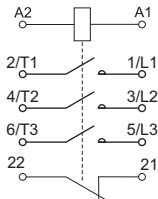
Рисунок 6 – Схема электрическая КМИе-10911 ÷ КМИе-23211 / Figure 6 – Electric diagram КМIе-10911 ÷ КМIе-23211 / 6 сурет – КМИе-10911 ÷ КМИе-23211 электрлі схемасы
