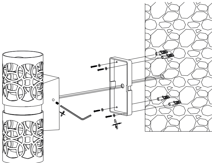
Рисунок 1 — Схема монтажа светильника
