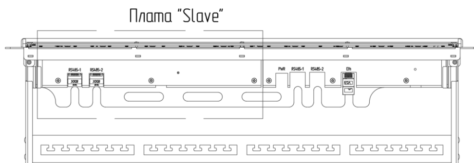
Расположение разъемов модуля (Slave) для интеллектуальной системы серии IQ Link
