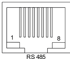
Рисунок 25 – Порт RS485
