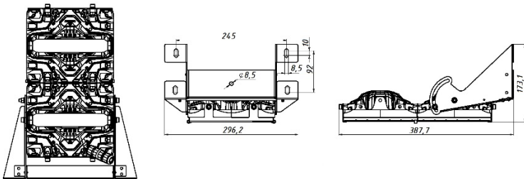
Рисунок 1 Общий вид светильника «L-pixel 2 banner» Поворотное крепление
