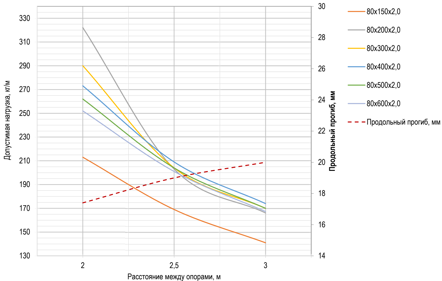
График нагрузок для лотков высотой 80 мм с толщиной стали 2 мм
