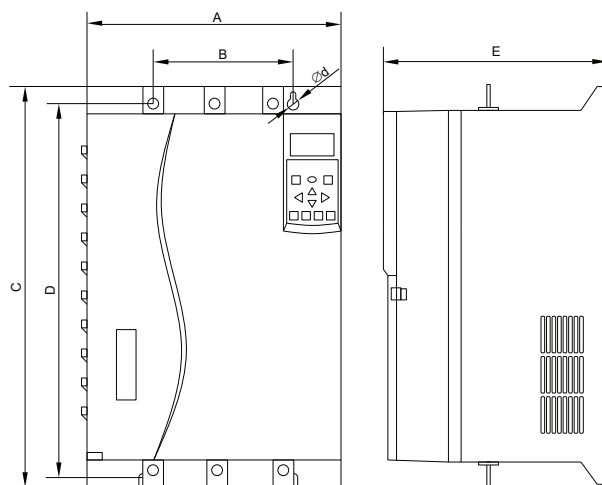
Рисунок 2.3 – Габаритные и установочные размеры УПП, габарит 2
