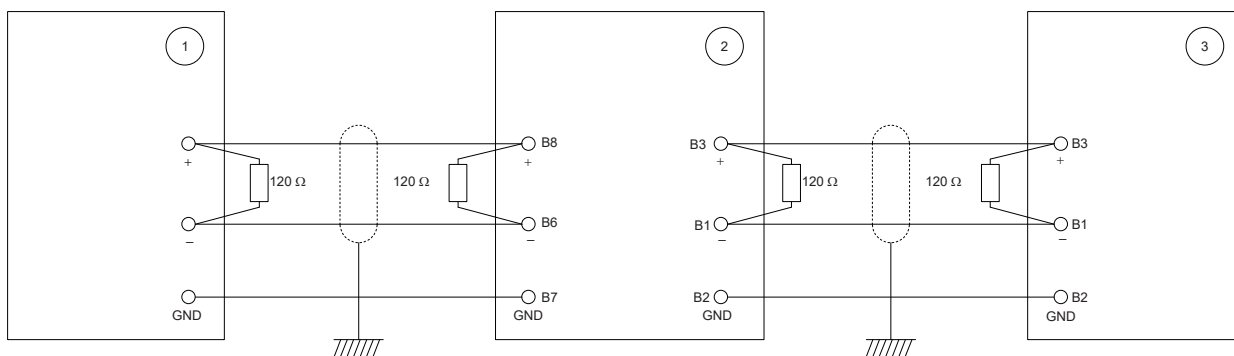
Рисунок Б.1 – Схема включения согласующих резисторов
