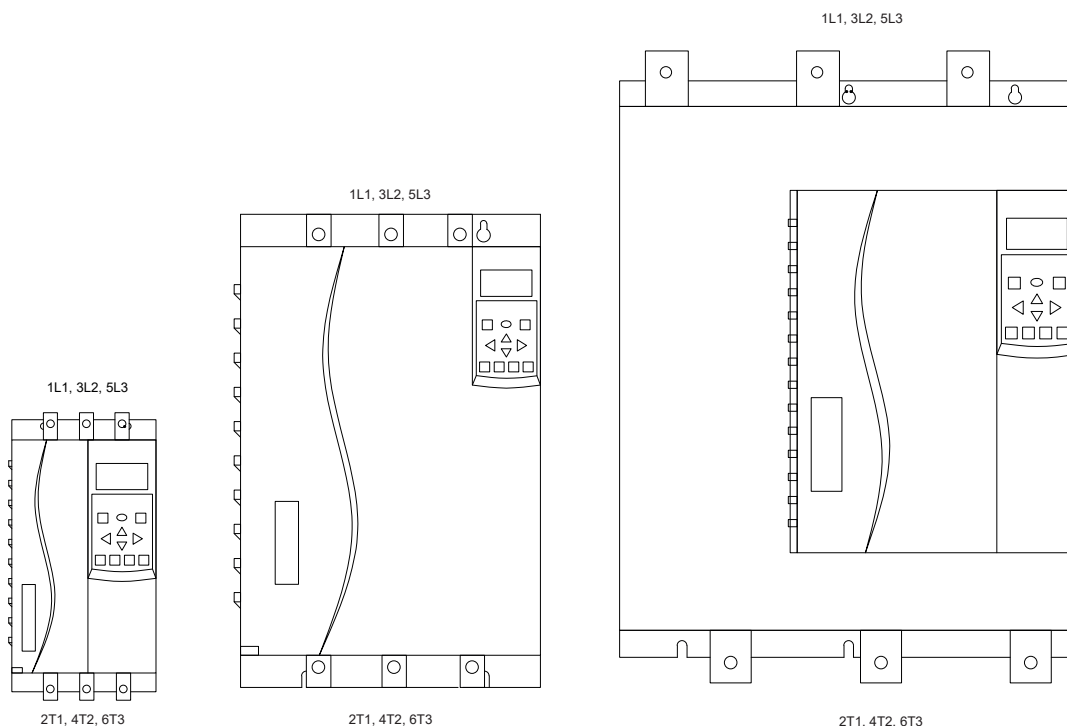
Рисунок 3.6 – Расположение силовых клемм
