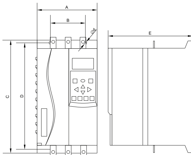
Рисунок 2.2 – Габаритные и установочные размеры УПП, габарит 1
