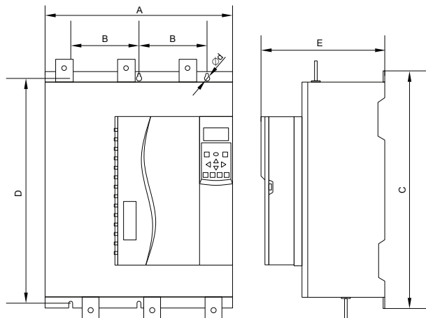
Рисунок 2.4 – Габаритные и установочные размеры УПП, габарит 3, 4
