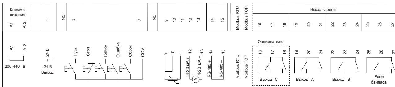
Рисунок 3.3 – Клеммы управления
