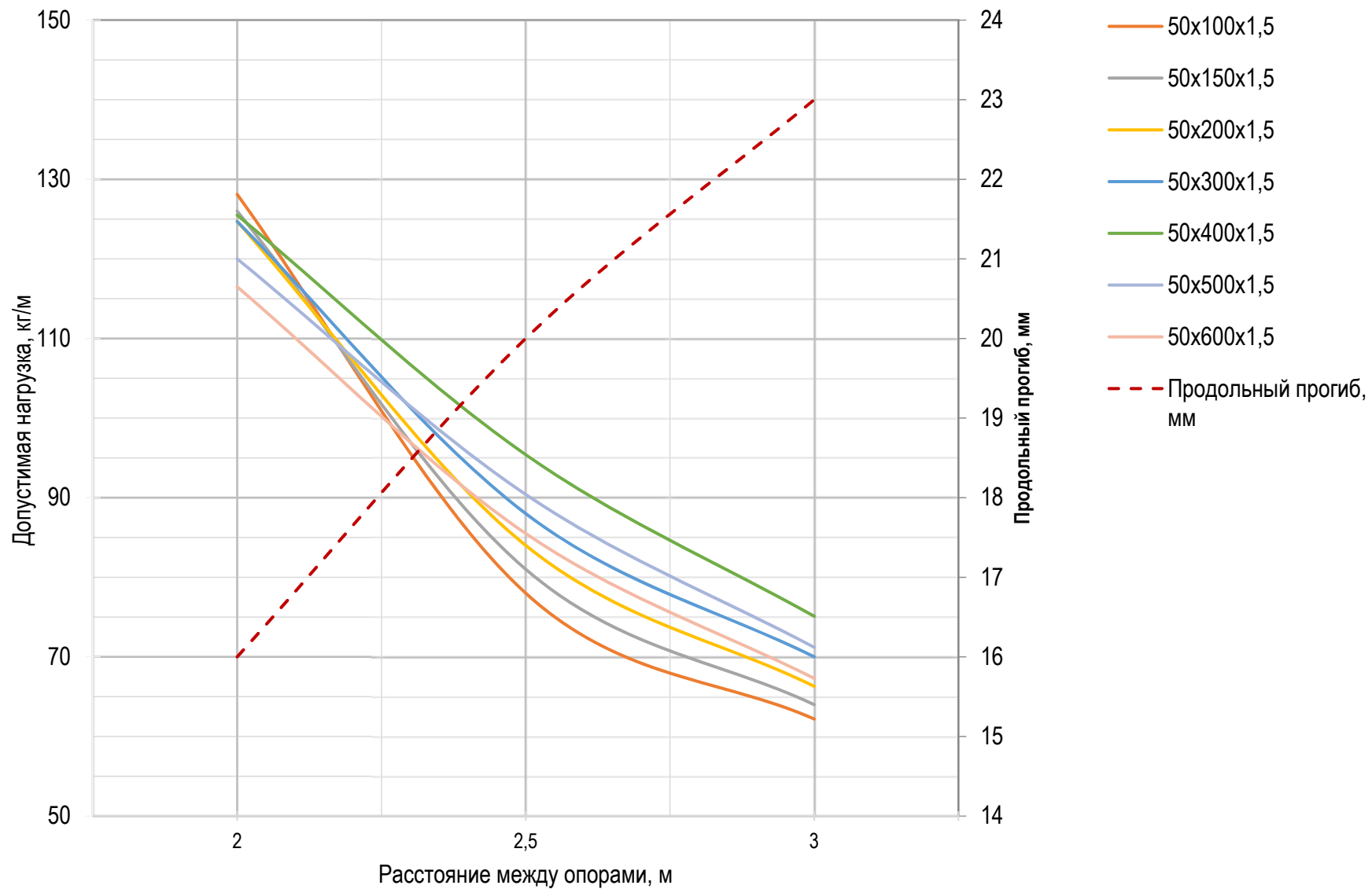
График нагрузок для лотков высотой 50 мм с толщиной стали 1,5 мм
