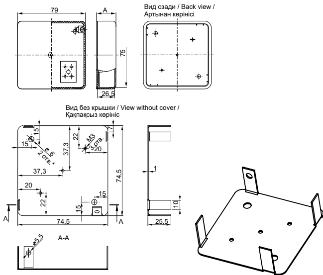
Рисунок / Figure / Сурет 1 – Коробка / Box / Қорап ПС 75×75×28
