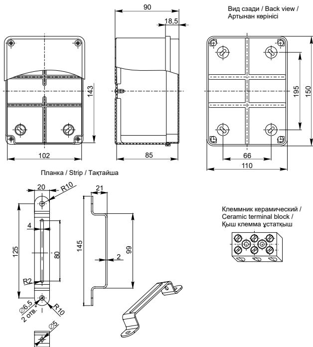
Рисунок / Figure / Сурет 3 – Коробка ПС 150×110×85 гладкие стенки / Вох ПС 150×110×85 smooth walls / ПС қорап 150×110×85 тегіс қабырғалары
