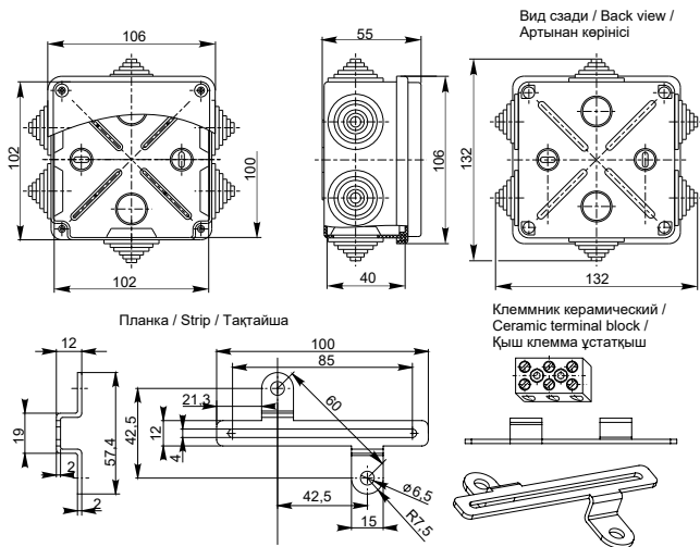
Рисунок / Figure / Сурет 4 – Коробка ПС 100×100×50 6 вводов / Box ПС 100×100×50 6 cable entries / ПС қорап 100×100×50 6 кірмесі
