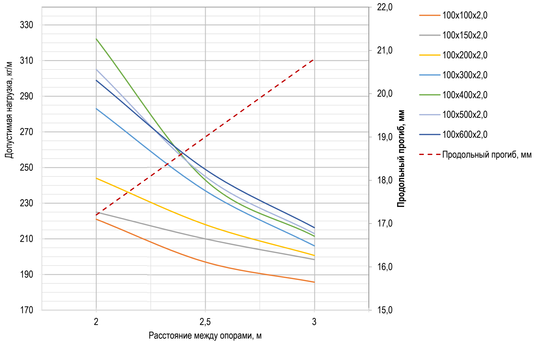
График нагрузок для лотков высотой 100 мм с толщиной стали 2 мм
