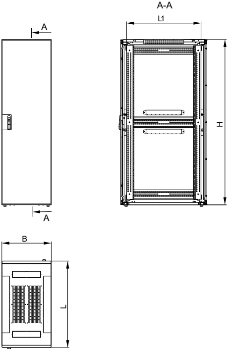
Рисунок 1 – Внешний вид шкафа / Figure 1 – Appearance of the cabinet / 1 сурет – Шкафтың сыртқы көрінісі
