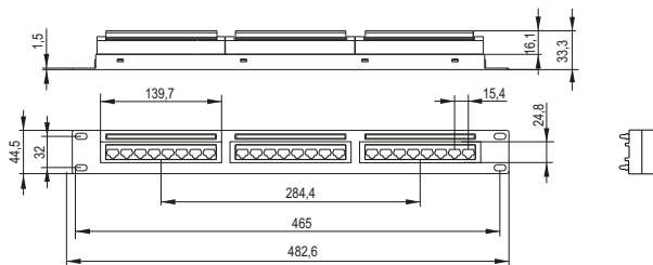
Рисунок/Figure 2 – PP24-1UC5EU-K05-G
