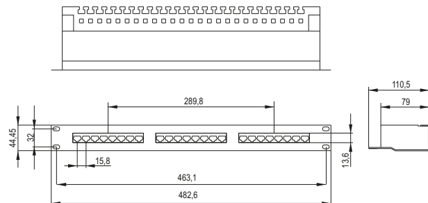
Рисунок/Figure 4 – PP24-1UC5EF-K05-G
