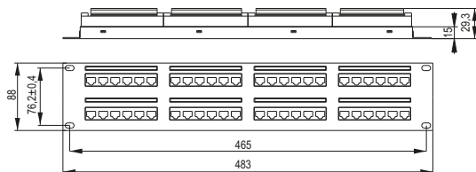
Рисунок/Figure 3 – PP48-2UC5EU-K05-G
