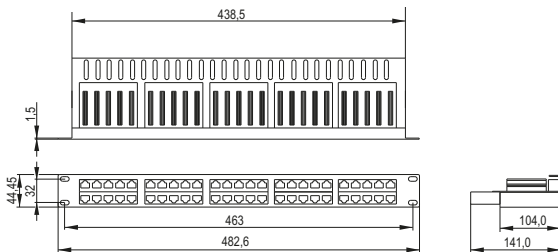
Рисунок/Figure 1 – PP50-1UC03U-K05-G
