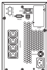
Внешний вид ИБП типа / Appearance of UPS of type / Типті ҰҚК сыртқы көрінісі EOT-0002KVA-1-004
