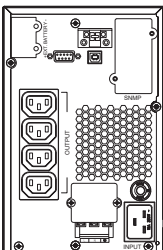
Внешний вид ИБП типа / Appearance of UPS of type / Типті ҰҚК сыртқы көрінісі EOT-0003KVA-1-L
