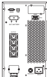
Внешний вид ИБП типа / Appearance of UPS of type / Типті ҮҚК сыртқы көрінісі EOT-0003KVA-1-006
