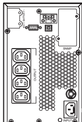
Внешний вид ИБП типа / Appearance of UPS of type / Типті ҰҚК сыртқы көрінісі EOT-0002KVA-1-L
