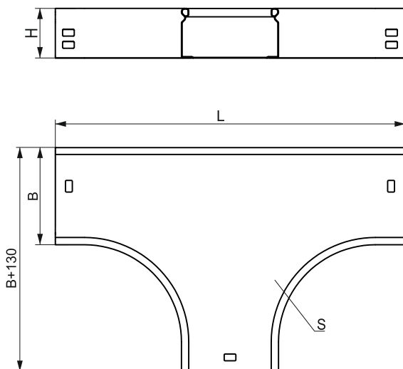
Рисунок 1 – Разветвитель Т-образный плавный серии ESCA
