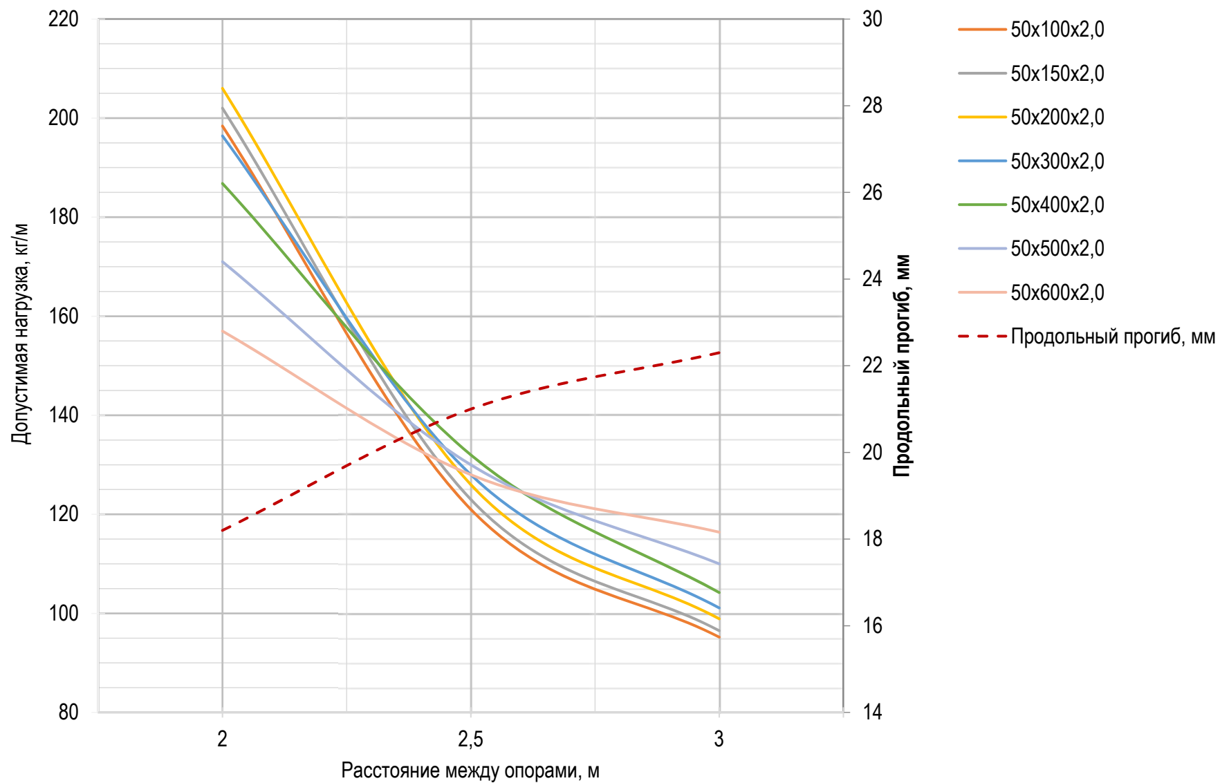
График нагрузок для лотков высотой 50 мм с толщиной стали 2 мм
