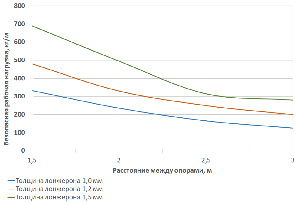
График нагрузок для лотков LESTA с высотой борта 150 мм
