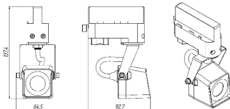
Рисунок 1 Светильник «L-mouse 3»
