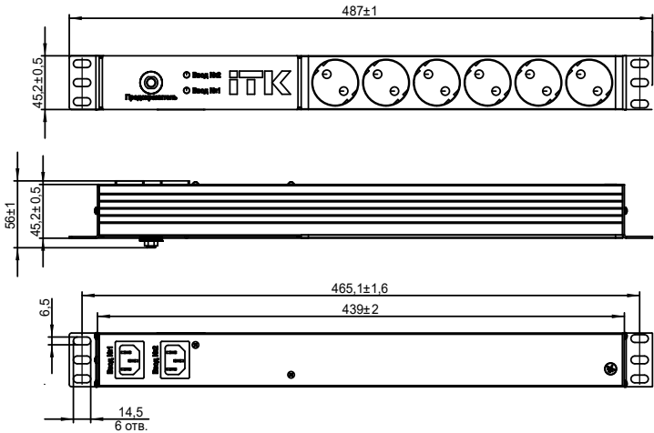
Рисунок / Figure 1 – Блок с АВР / A block with AVR
