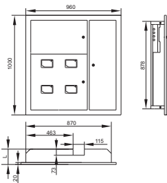
Рисунок / Figure / Сурет 1 – Корпус на 2–6 квартир / Enclosure for 2–6 apartments / 2–6 пәтерге арналған корпус
