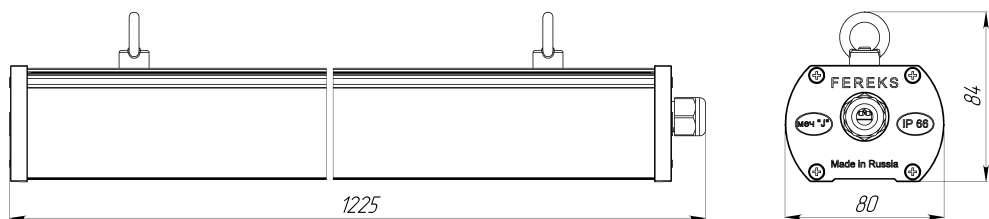
Рисунок 1. Светильник ДСО
