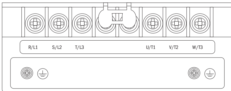
Схема 2.3. Подключение клемм силовых цепей 1PH 220 В 1,5 и 2,2 кВт 3PH 380 В 0,75+2,2 кВт
